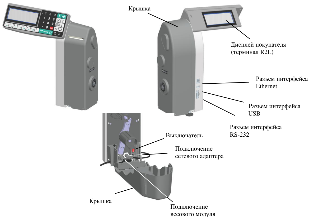
Рис. 2.1 – Общий вид терминалов RL и R2L
