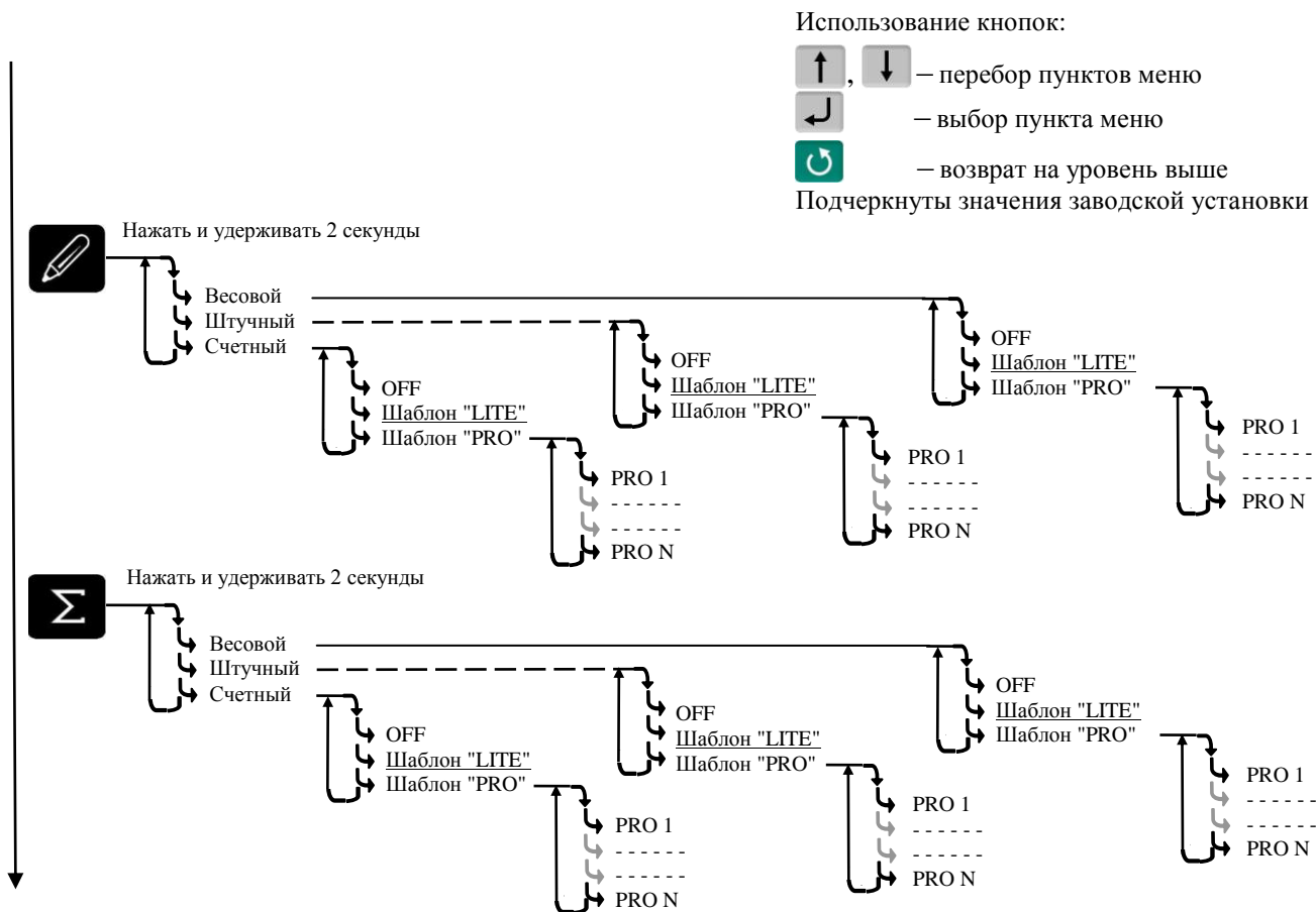
Рис. 4.2 – Схема установки шаблонов печати
