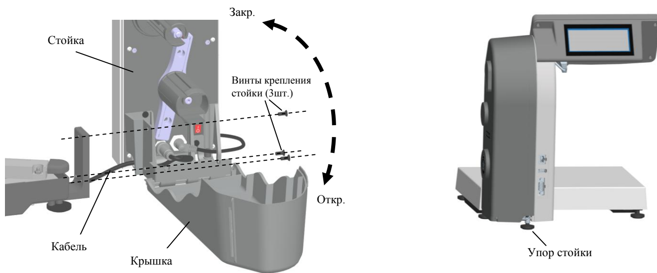
Рис. 2.3 – Крепление терминала в весах МК-RL, МК-R2L
