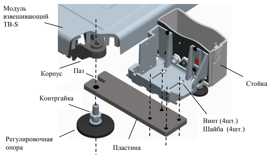
Рис. 2.4 – Крепление терминала к взвешивающему модулю ТВ-S
